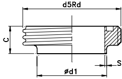
MACHO SOLDAR SMS WELDING MALE SMS ШТУЦЕР РЕЗЬБОВОЙ SMS ПОД СВАРКУ
