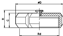
TUERCA CIEGA CON PIVOTE BLIND NUT WITH BOSS ГАЙКА-ЗАГЛУШКА С БОЫШКОЙ
