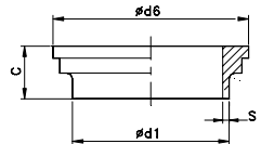
CASQUILLO SOLDAR SMS WELDING LINER SMS ШТУЦЕР ПОД СВАРКУ SMS
