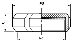
TUERCA CIEGA SMS BLIND NUT SMS ГАЙКА-ЗАГЛУШКА SMS
