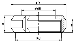
TUERCA SMS NUT SMS ГАЙКА SMS
