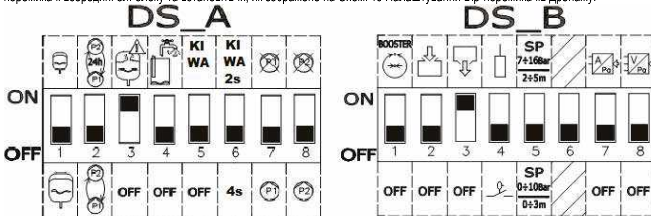
Схема 40: Налаштування Dip-перемикачів Дренажу
