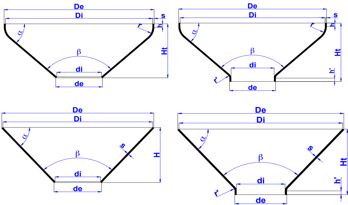
Концентрическое днище / Конический переход
