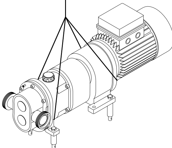
рис 4.1: переноска насоса.
